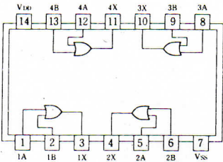
4071B
