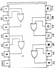
7432
