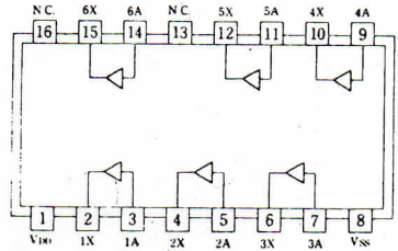
4050UB
