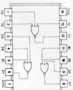
7427
