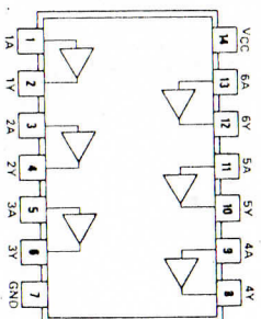
7407
