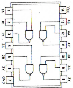
7400
