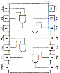
7408
