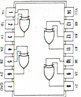
7486
