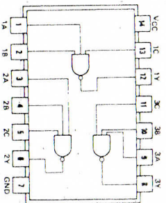
7410
