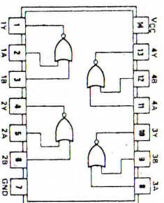
7402
