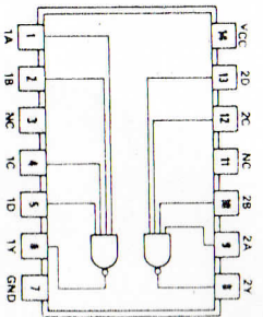
7420
