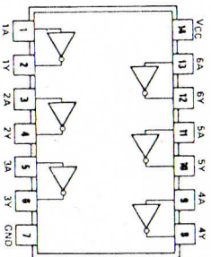
7404
