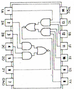
74LS51
