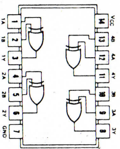
74136
