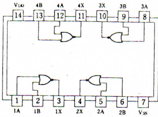
4001B
