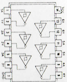
7414
