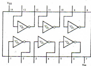
40106B
