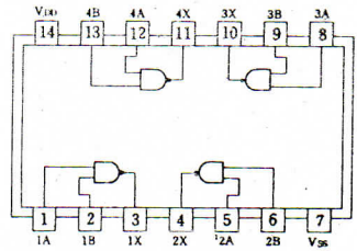
4011B
